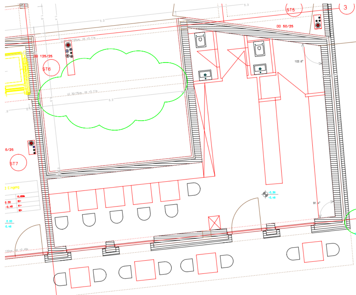
Grundriss Gewerbe 2 Erdgeschoss
